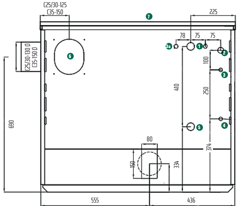
Premiumline Ansicht hinten , RECHTE* Ausführung
