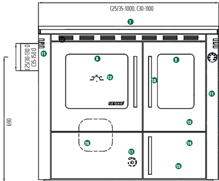
Premiumline Ansicht vorne , LINKE* Ausführung
